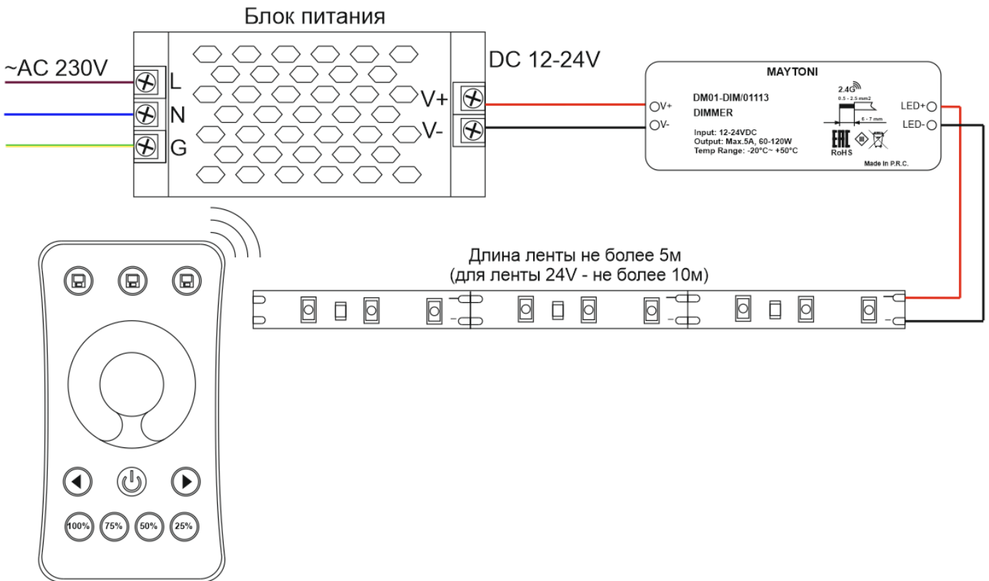
Рис. 1 схема подключения диммера
